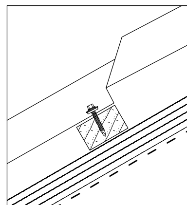
Надлъжен разрез
